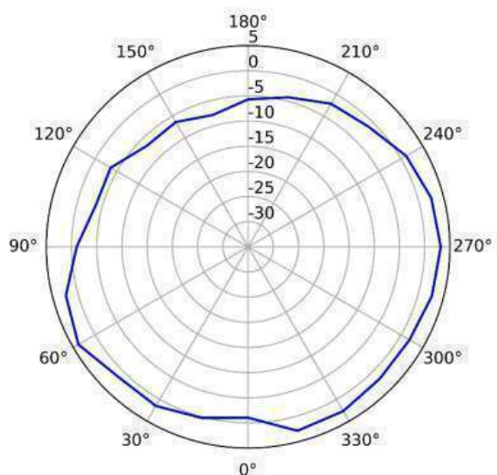
5GHz (Vertical)
