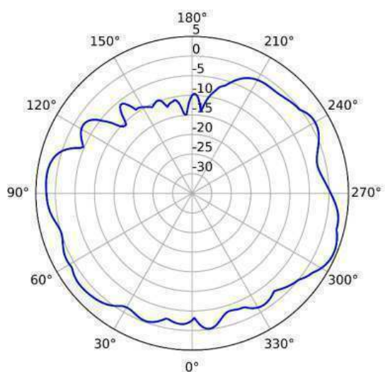
6GHz (Vertical)
